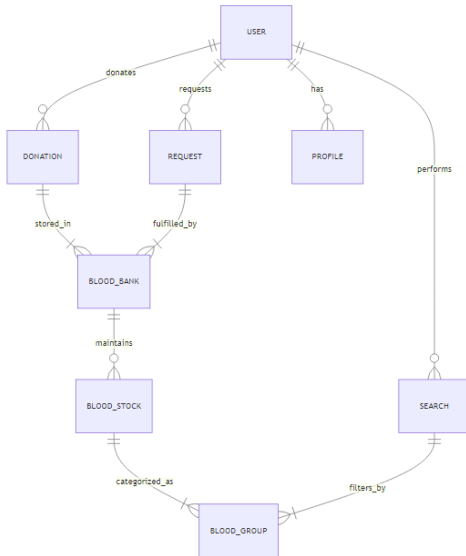
Figure 2.1 ER Diagram
